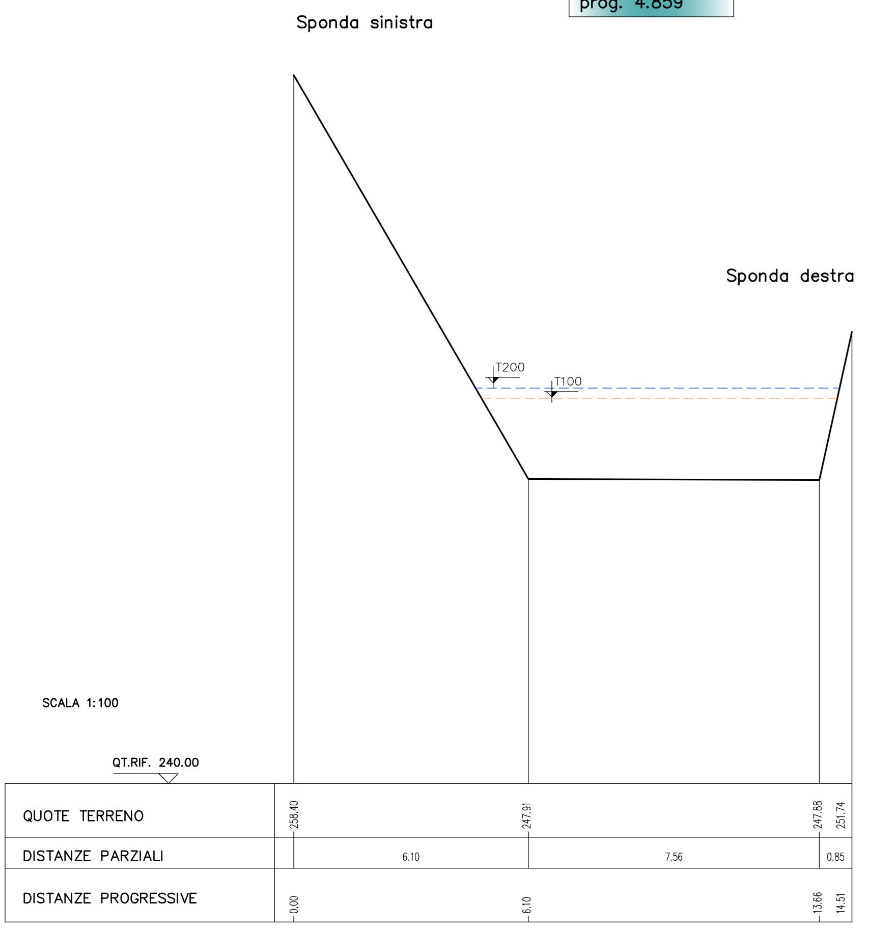
Sezione 33.2 prog. 4.859
