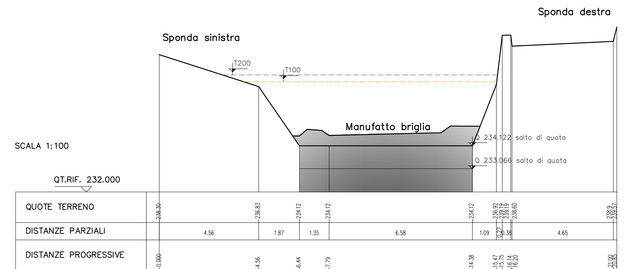
Sezione 36 prog. 5.373
