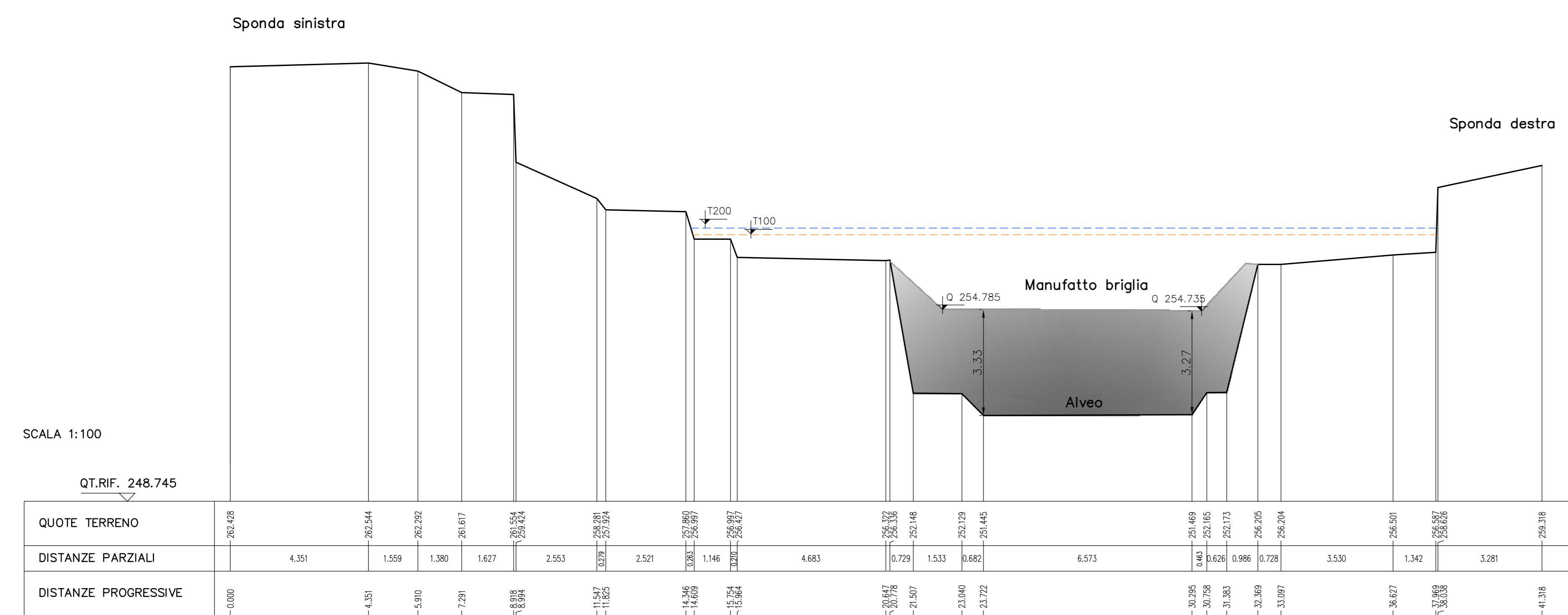
Sezione 33.2 prog. 4.859
